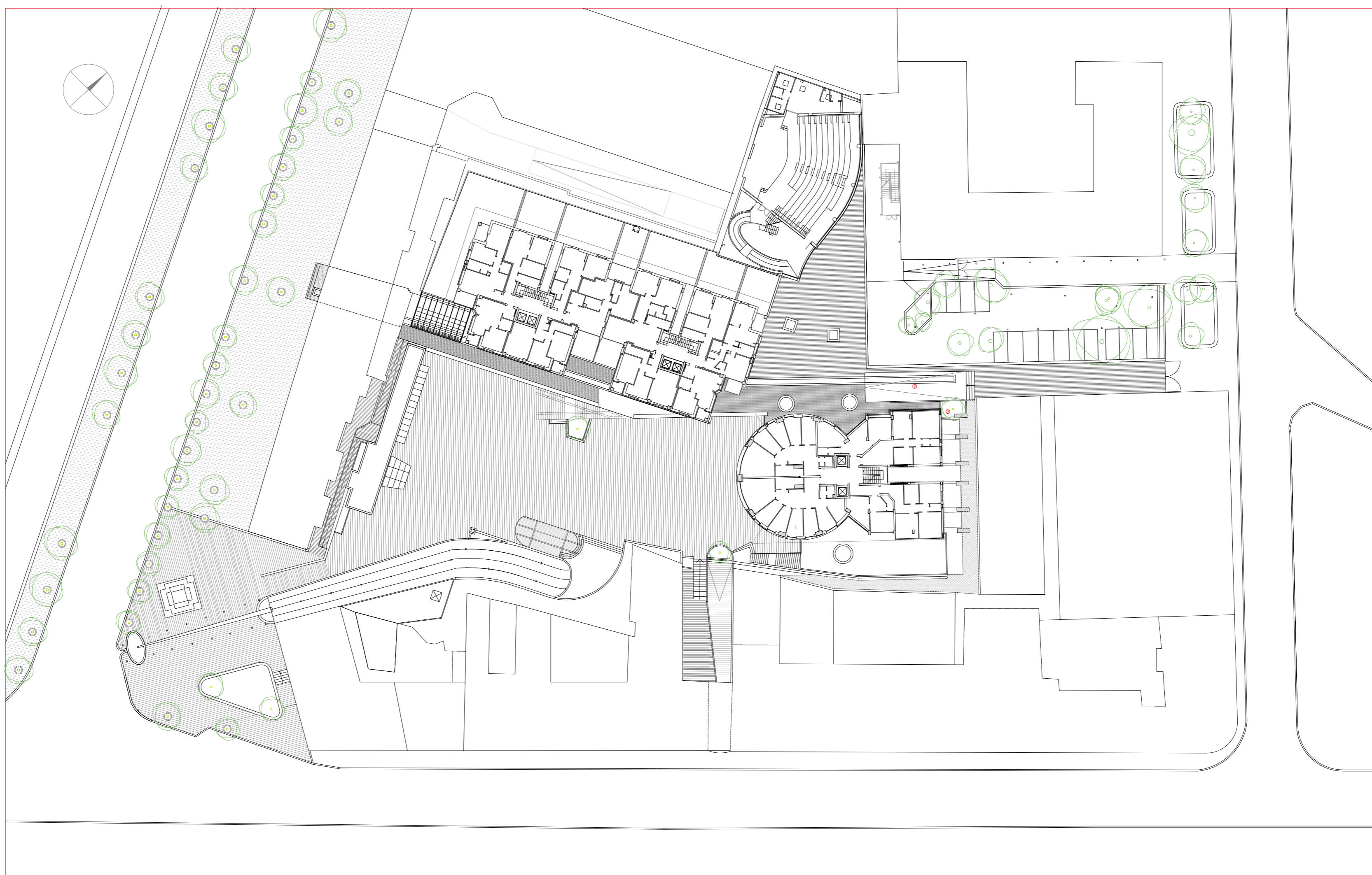
Pianta 1° livello residenziale direzionale
