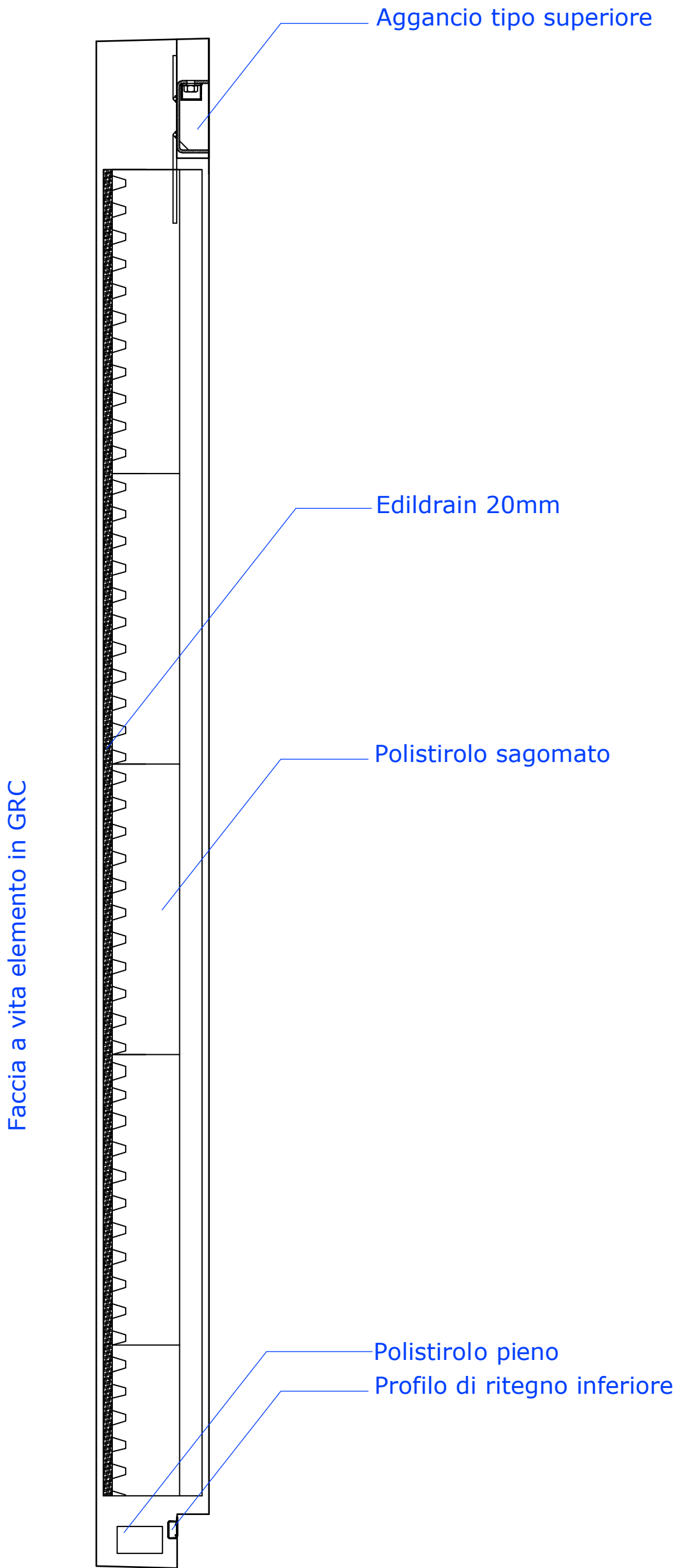
SEZIONE TIPO PANNELLO GRC
